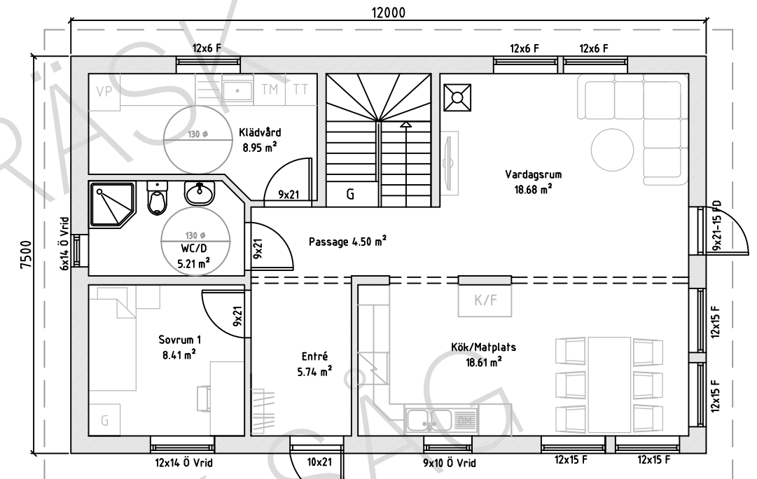
NEDRE PLAN
