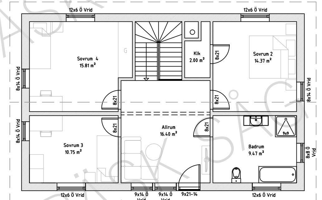
ÖVRE PLAN
